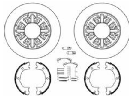
Kit complet de frein de parking
