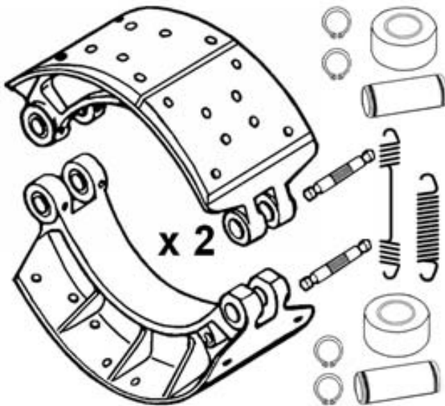
MAXIKIT FRICTION
